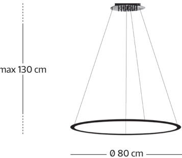
art. KLAQ S 80 telaio altezza regolabile / frame with adjustable height max 12 cablaggi CP 200 / max 12 cables CP 200
