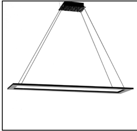
KLAQ/S 120 largh. 120 lungh. 40 h. 130 regolabile
